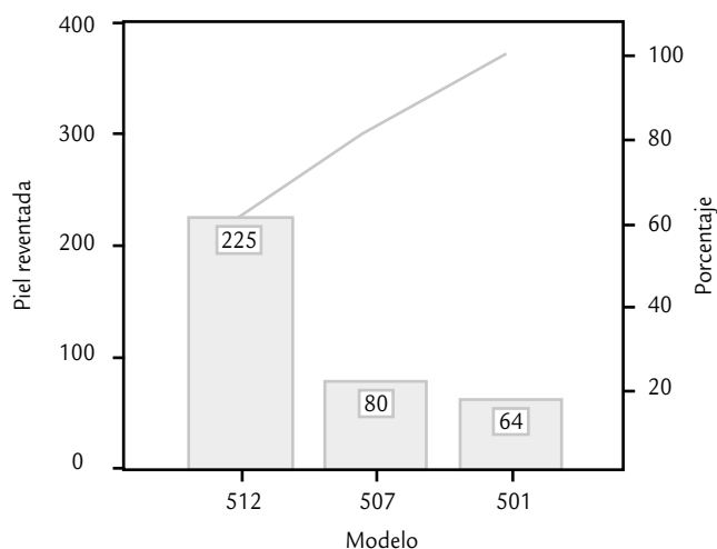
FIGURA 6.2 Pareto para causas: defecto principal por modelo de botas.
